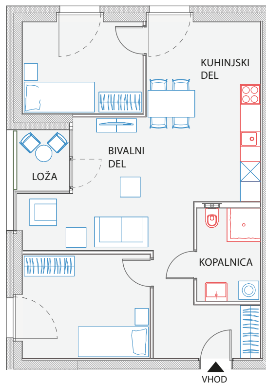
Primer stanovanja velikosti 70 m 2
