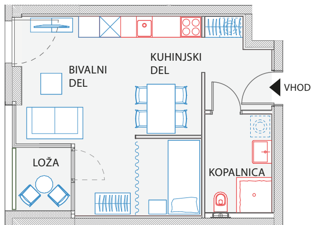
Primer stanovanja velikosti 56 m 2
